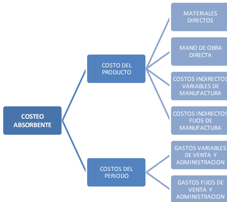
Gráfico 4.1 Costeo Absorbente
