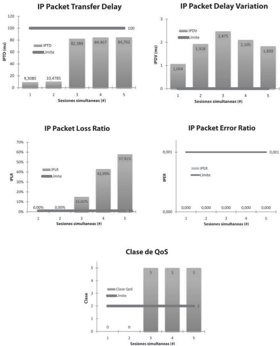
Figura 28. Medidas de QoS para sesiones de juego en línea
