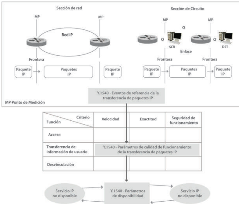
Figura 1. Alcance de la Recomendación ITU-T Y.1540(2: 2)
