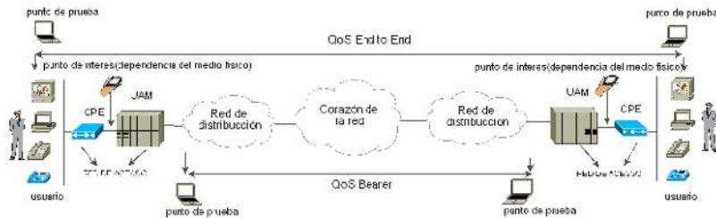
Figura 13. Tipos de medición de QoS(5)
