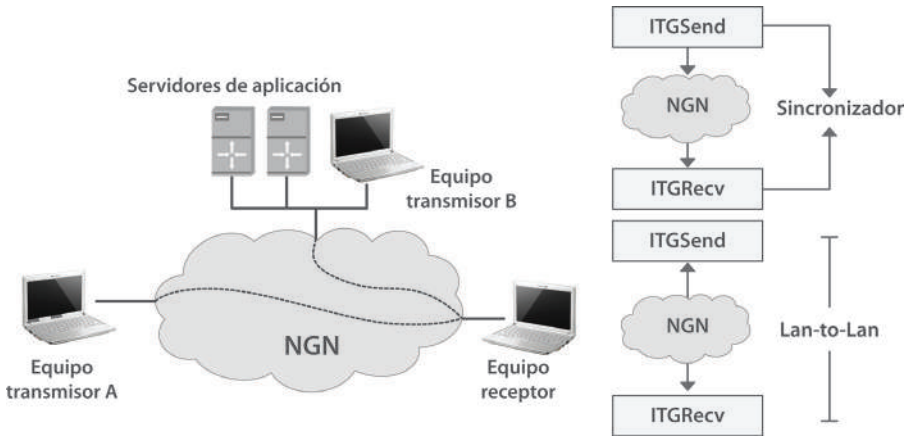
Figura 18. Forma de operación del D-ITG(9)
