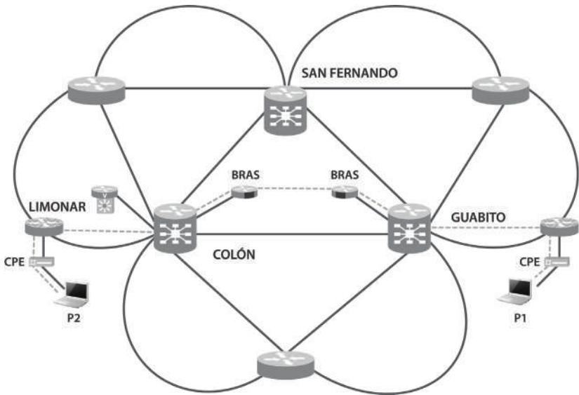
Figura 22. Red utilizada para realizar las mediciones de prueba (Fuente: Emcali)
