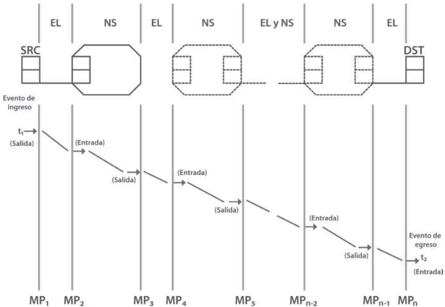
Figura 6. Eventos de retardo de transferencia de paquetes IP. Transferencia ‘extremo a extremo’ de un paquete IP(2: 17)
