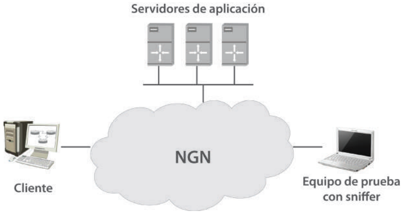
Figura 17. Captura de protocolos y estadísticas de transmisión de las aplicaciones a las que se medirá la QoS
