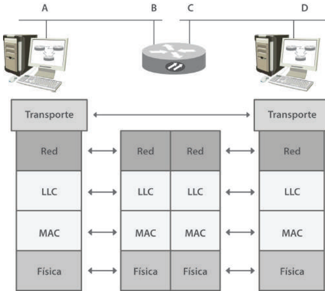
Figura 16. Funcionamiento a nivel de protocolos del D-ITG(9)
