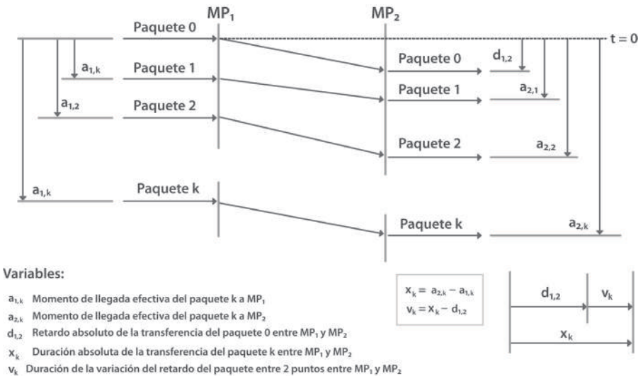
Figura 7. Variación del retardo de paquetes IP entre dos puntos.(2: 18)
