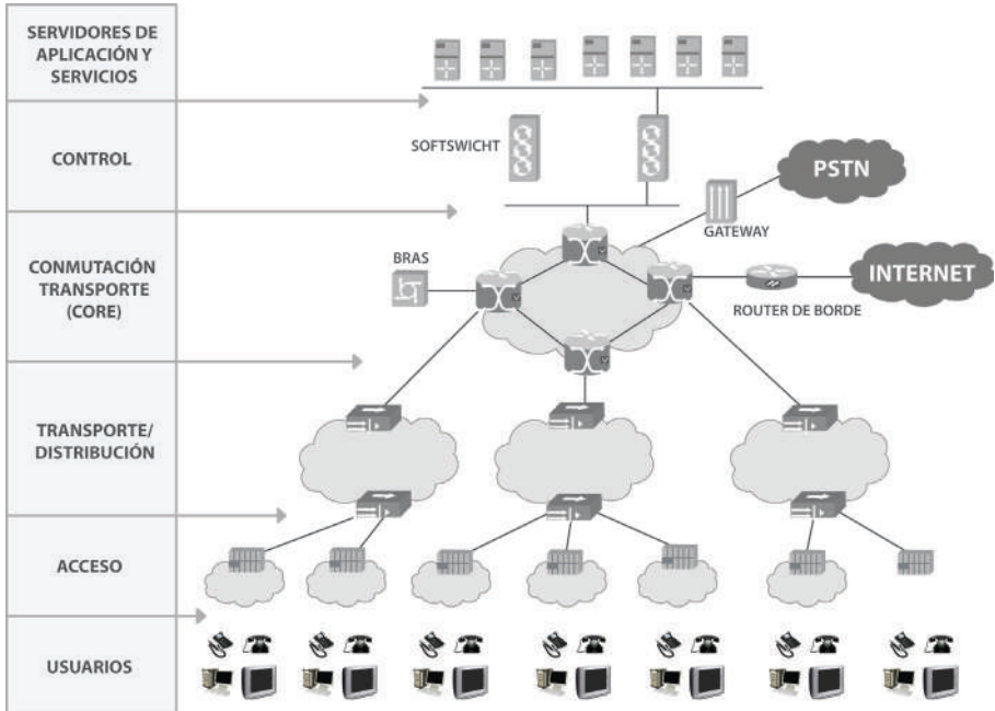
Figura 11. Esquema General de la NGN de EMCALI (Fuente:Emcali)
