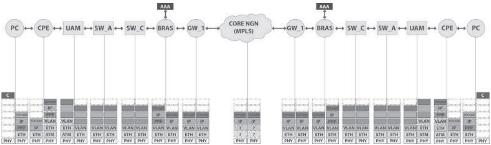
Figura 24. Protocolos que intervienen en una comunicación extremo a extremo en la NGN de Emcali (Fuente: Emcali)
