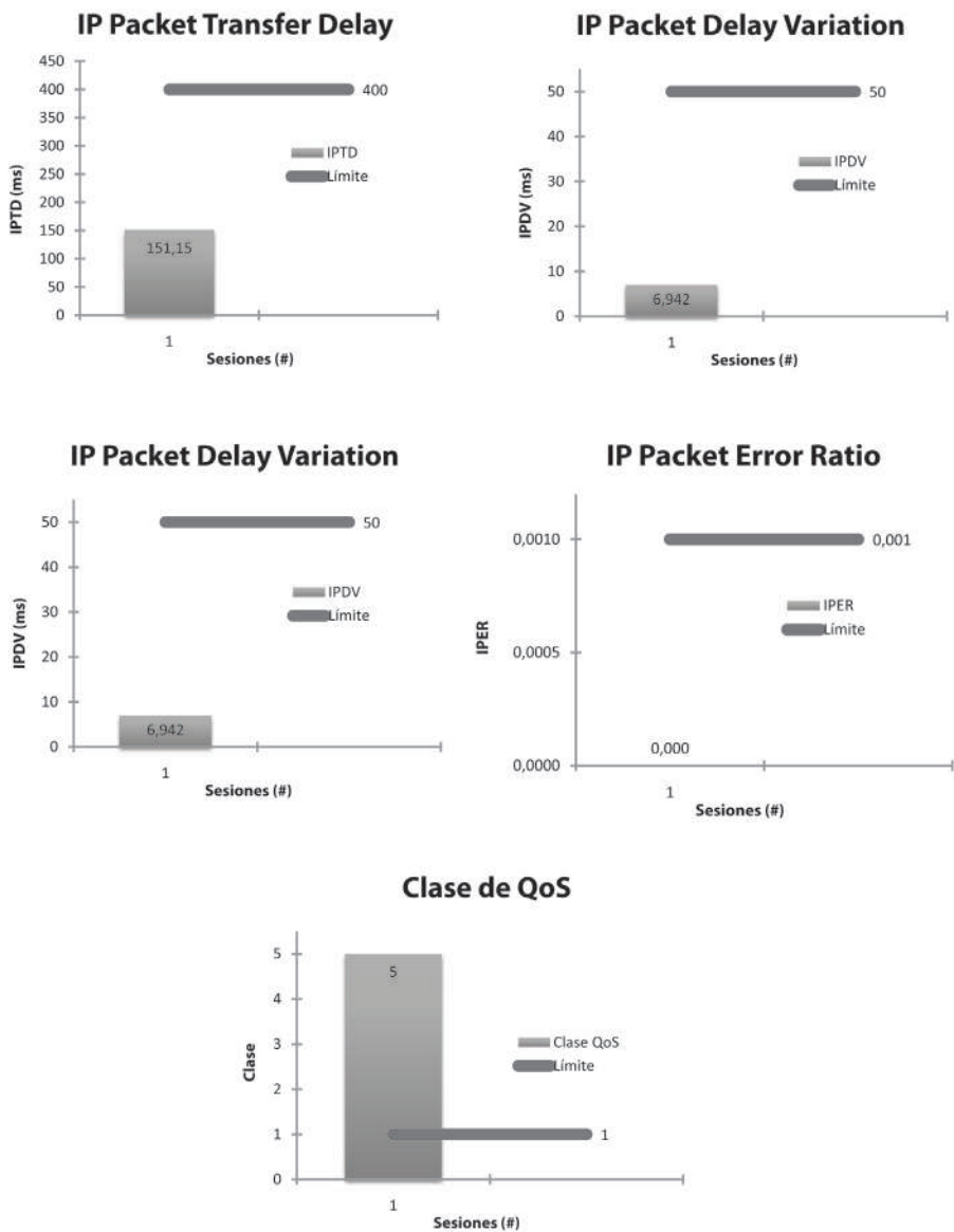
Figura 25. Medidas de QoS para IPTV
