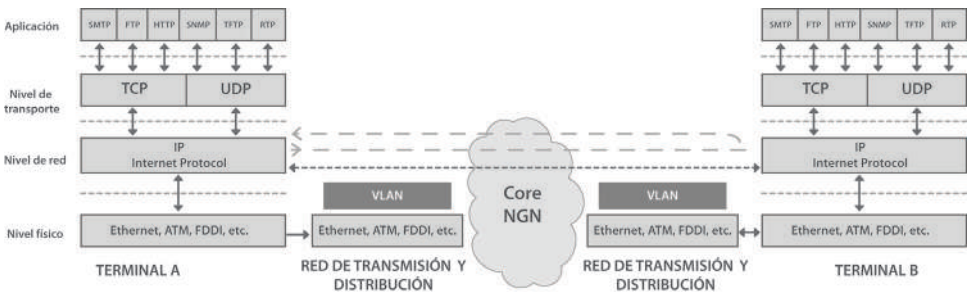
Figura 19. Operación del D-ITG ante la presencia de conmutación a nivel 2 (9)
