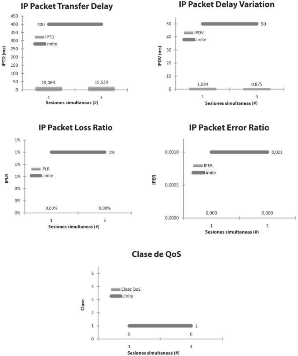
Figura 26. Medidas de QoS para difusión de audio
