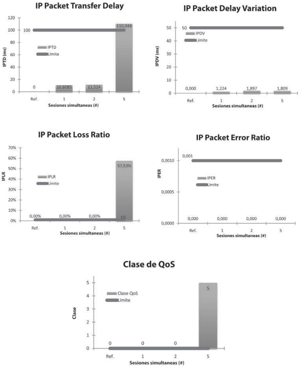
Figura 27. Medidas de QoS para llamadas telefónicas IP
