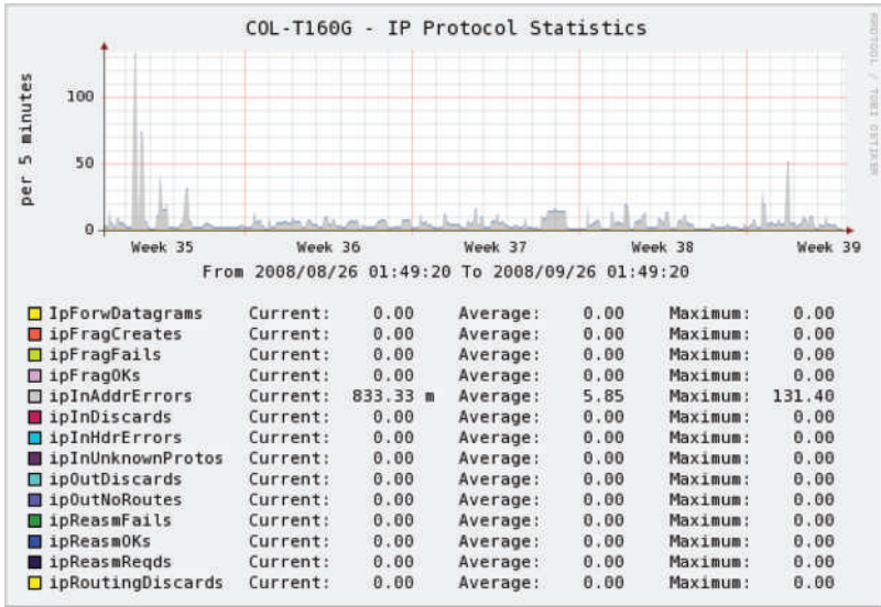
Figura 23. Estadísticas de carga IP de uno de los equipos del Core de la red en el momento de realización de las pruebas.
