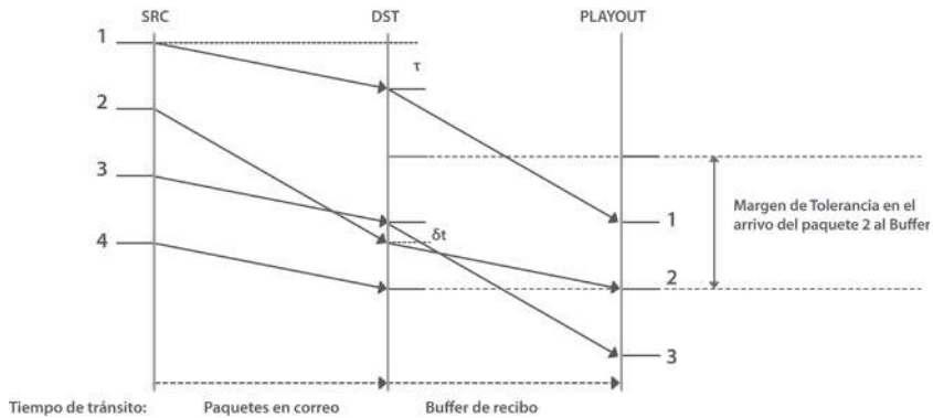
Figura 8. Ilustración del orden de arribo(2: 31)
