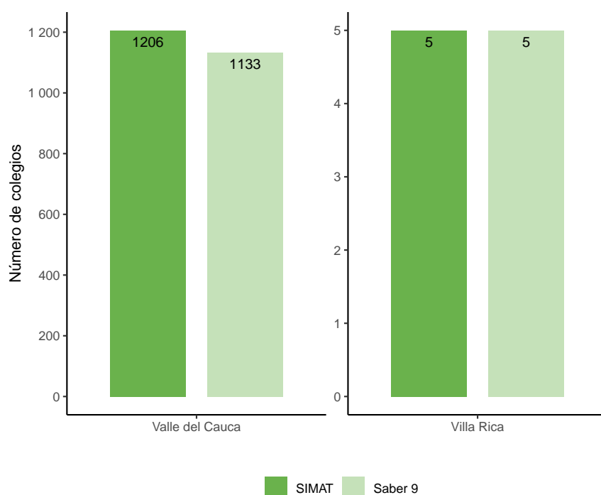
Figura 3.3: Número de colegios con estudiantes tomando el examen Saber 9 y número de colegios que ofrecen formación en el grado 9 en Valle del Cauca y Villa Rica en 2017
